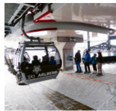
Der Auenfeldjet verbindet die Skigebiete Warth-Schröcken und Lech. In Lech fädelt sich die 10er-Kabinen auf das Seil einer bestehenden Sesselbahn ein.
